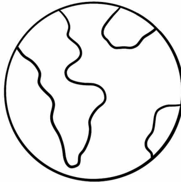
TERRA
