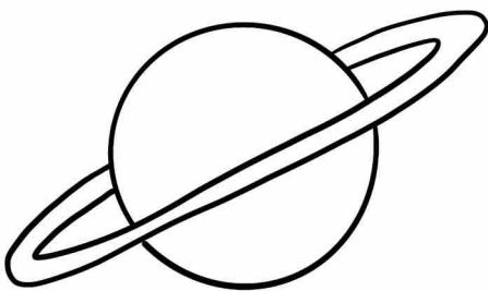
URANO
