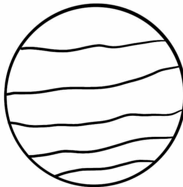
VENERE
