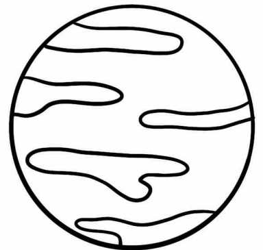
NETTUNO
