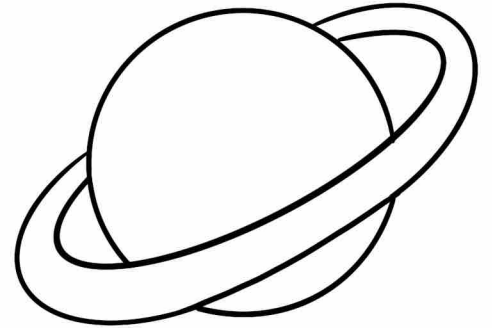
SATURNO
