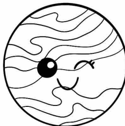
MERCURIO
