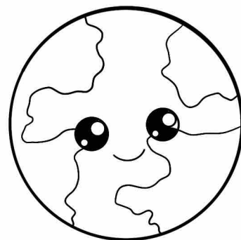
TERRA
