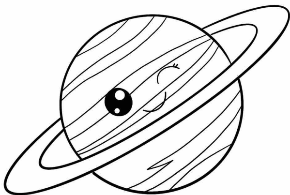
SATURNO
