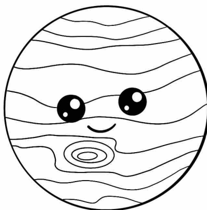
GIOVE
